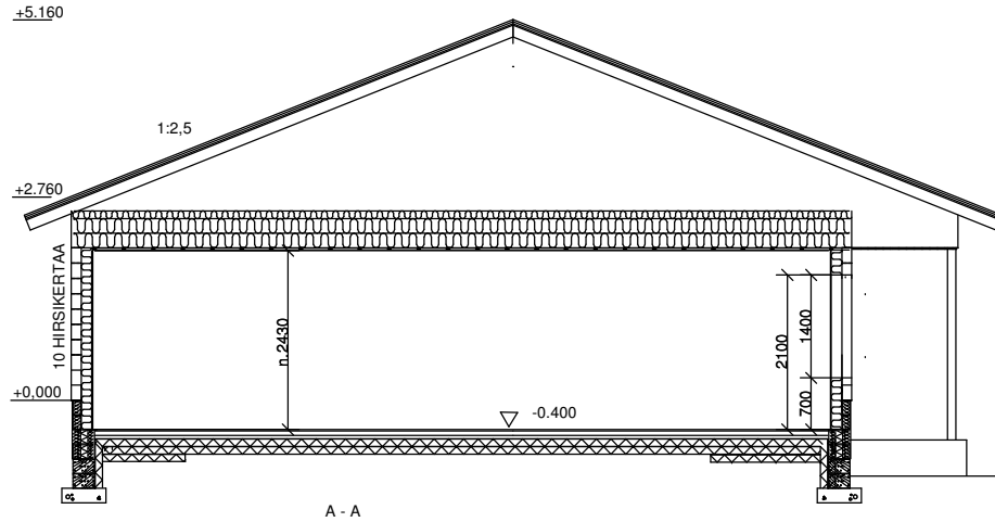
A - A
