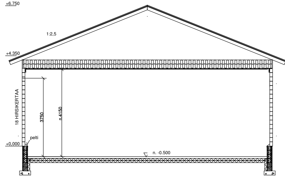
B - B
